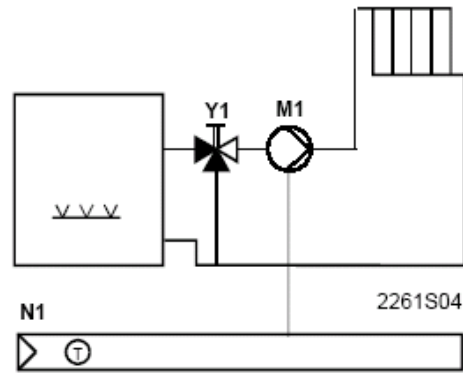
手动混合阀预控制的循环泵
